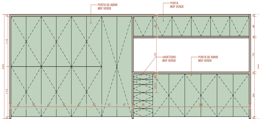
ARMARIO 01 - OP01 ESC. 1:25
